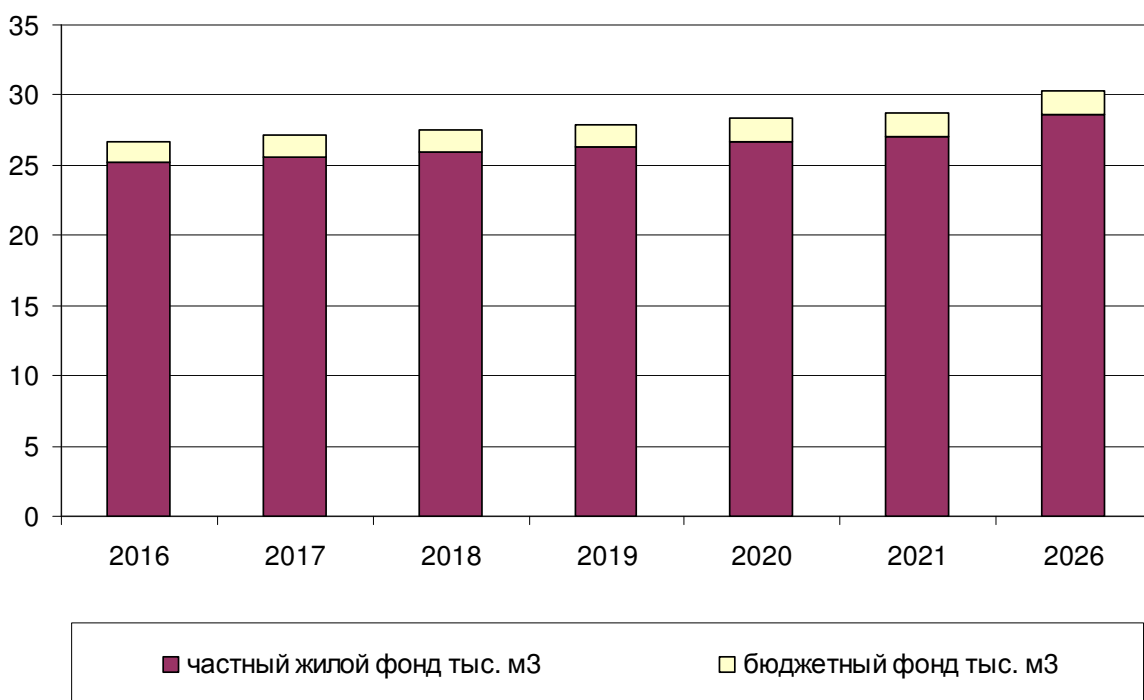
Рисунок 13 – Диаграмма перспективного баланса подачи и реализации воды по структурным составляющим
