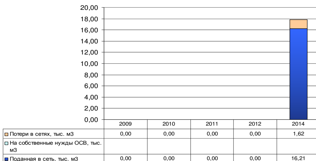
Рисунок 7 – Составляющие подачи и распределения воды в системе водоснабжения за 2014 г.
