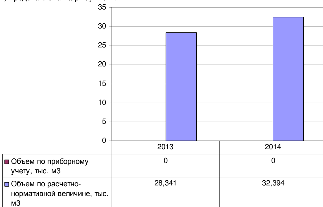
Рисунок 17 – Динамика изменения объемов потребления воды по фактическим и расчетным данным за период с 2013 по 2014 гг.
