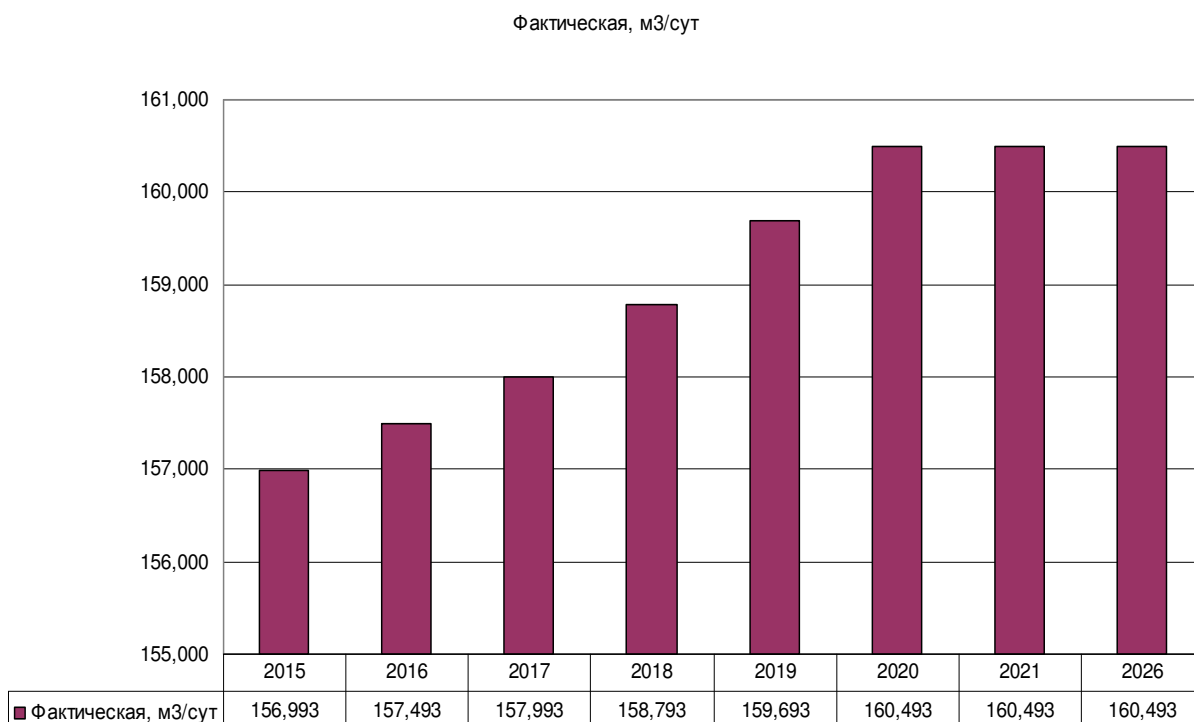
Рисунок 23 – Прогноз перспективного среднесуточного потребления воды МО «Кулюшевское»
