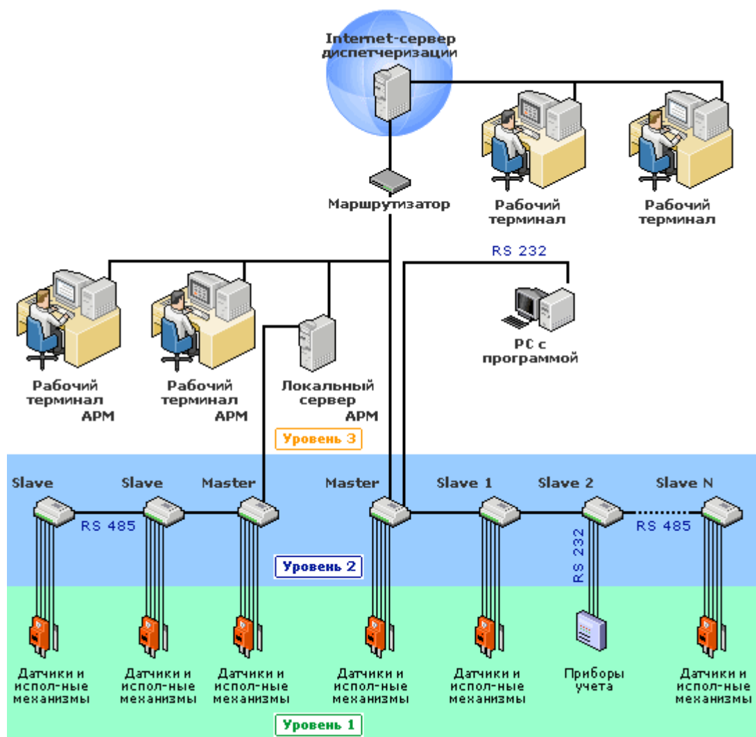
Рисунок 25 – Схема уровней системы АСУ ТП
