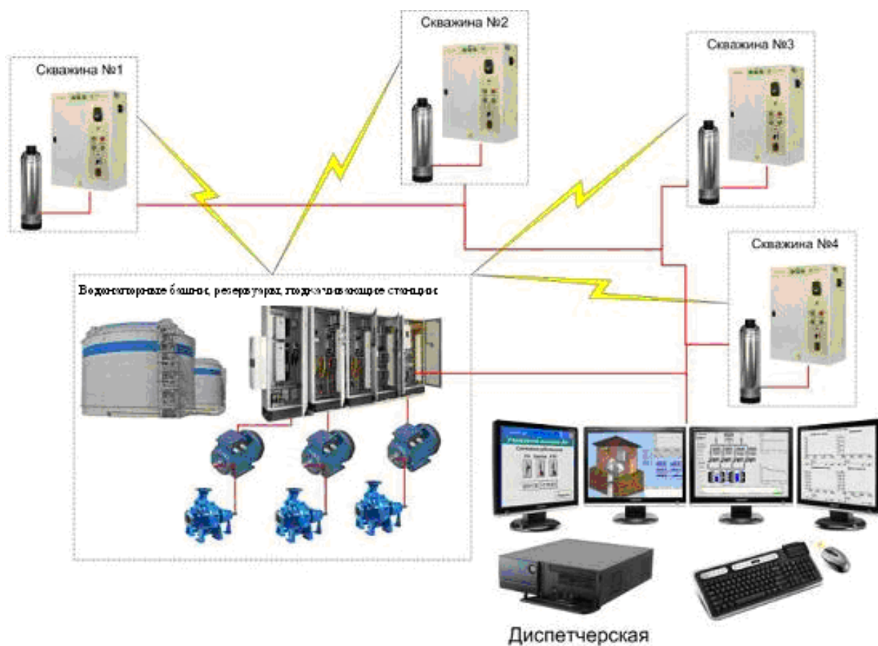
Рисунок 24 – Схема автоматизации, диспетчеризации и управления
