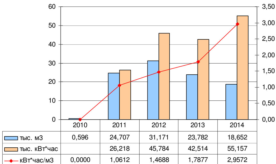
Рисунок 5 – Динамика изменения объемов потребления энергоресурсов скважиной с. Галаново №934 ул. Ушакова за период с 2010-2014 гг.
