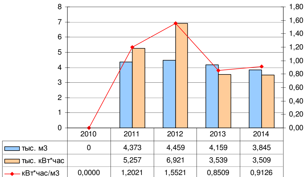
Рисунок 9 – Динамика изменения объемов потребления энергоресурсов скважиной №1911 д. Сухарево за период с 2010-2014 гг.
