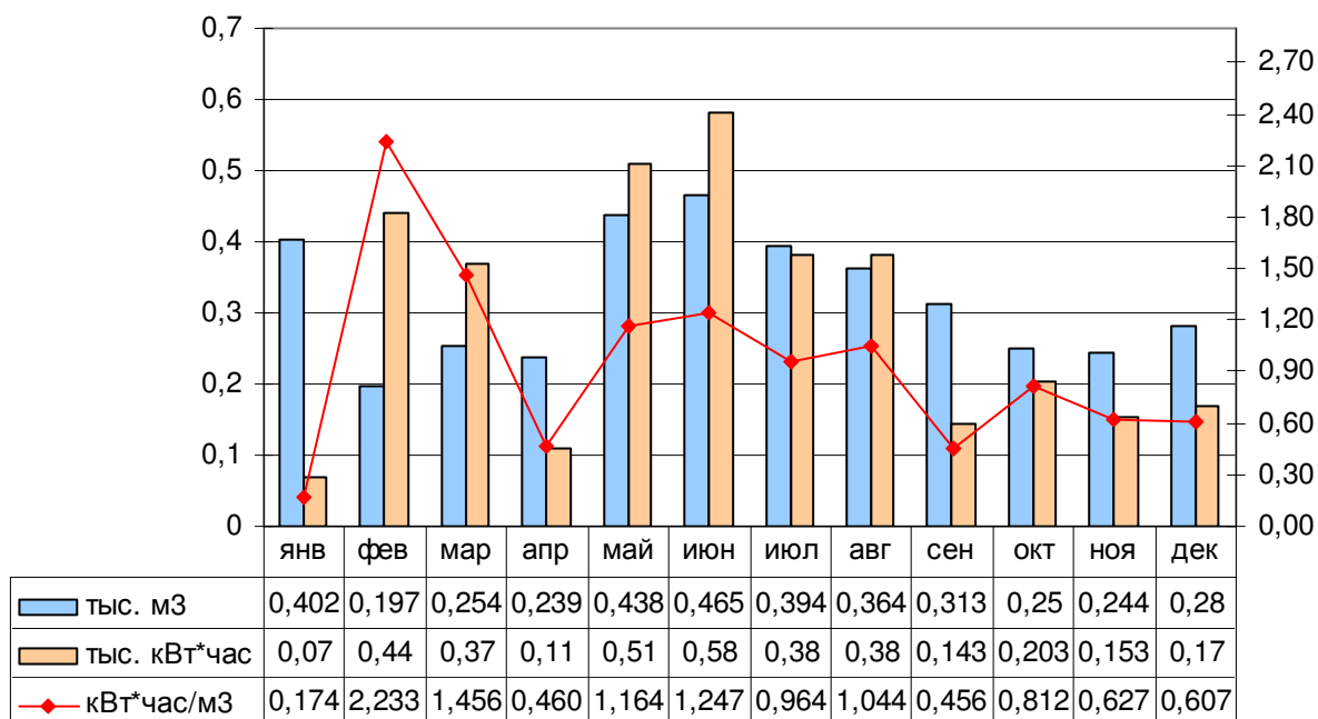
Рисунок 10 – Динамика сезонного изменения объемов потребления электроэнергии скважиной №1911 д. Сухарево за 2014 г.
