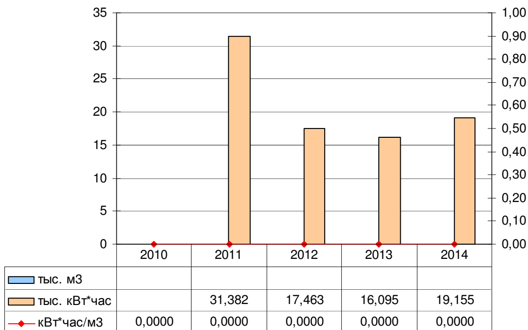
Рисунок 7 – Динамика изменения объемов потребления энергоресурсов скважиной с.Галаново №2968 ул. Камская за период с 2010-2014 гг.
