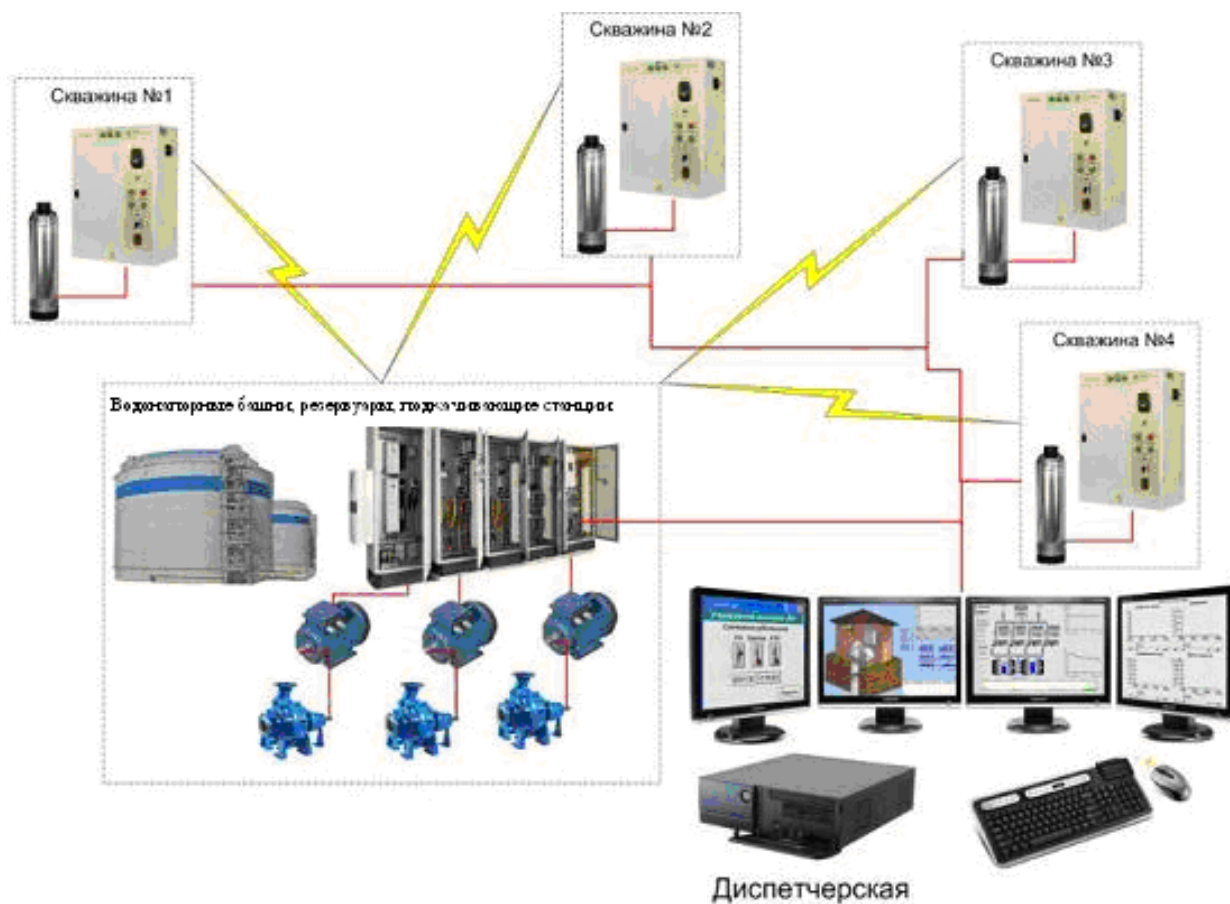
Рисунок 28 – Схема автоматизации, диспетчеризации и управления
