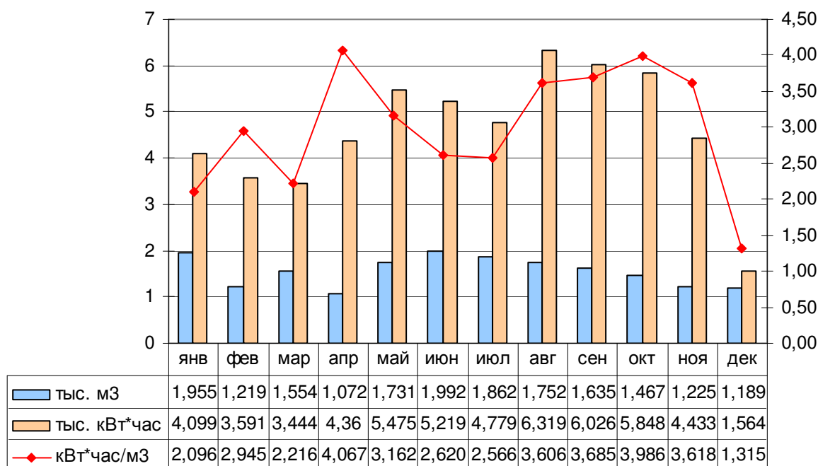
Рисунок 6 – Динамика сезонного изменения объемов потребления электроэнергии скважиной с. Галаново №934 ул. Ушакова за 2014 г.
