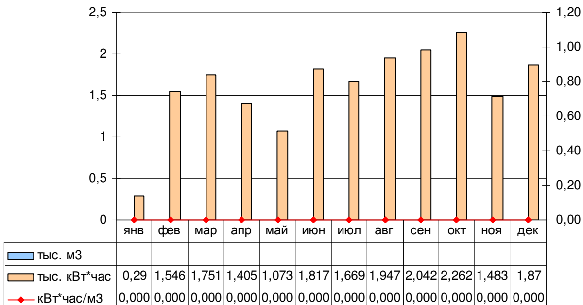
Рисунок 8 – Динамика сезонного изменения объемов потребления электроэнергии скважиной с.Галаново №2968 ул. Камская за 2014 г.
