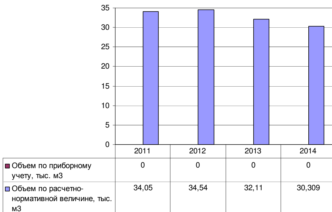
Рисунок 16 – Динамика изменения объемов потребления воды по фактическим и расчетным данным за период с 2011 по 2014 гг.
