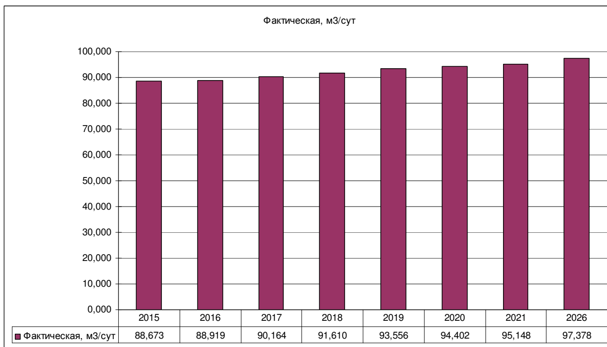
Рисунок 21 – Прогноз перспективного среднесуточного потребления воды МО «Боярское»
