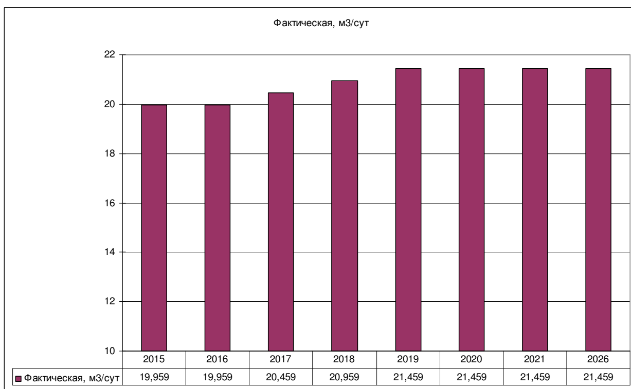
Рисунок 20 – Прогноз перспективного среднесуточного потребления воды д. Кухтино
