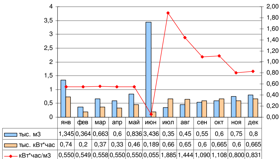
Рисунок 6 – Динамика сезонного изменения объемов потребления электроэнергии скважинами МО «Боярское» за 2014 г.
