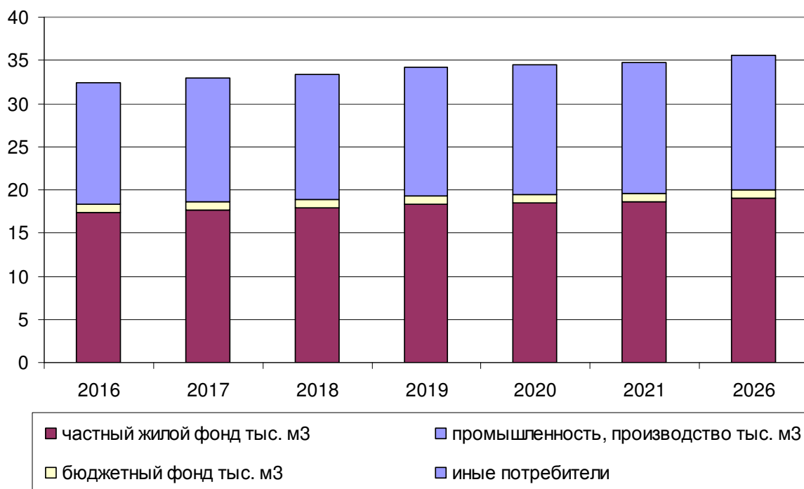
Рисунок 18 – Диаграмма перспективного баланса подачи и реализации воды по структурным составляющим
