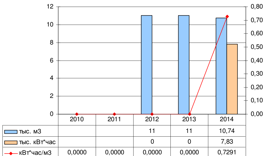
Рисунок 5 – Динамика изменения объемов потребления энергоресурсов скважинами МО «Боярское» за период с 2010-2014 гг.
